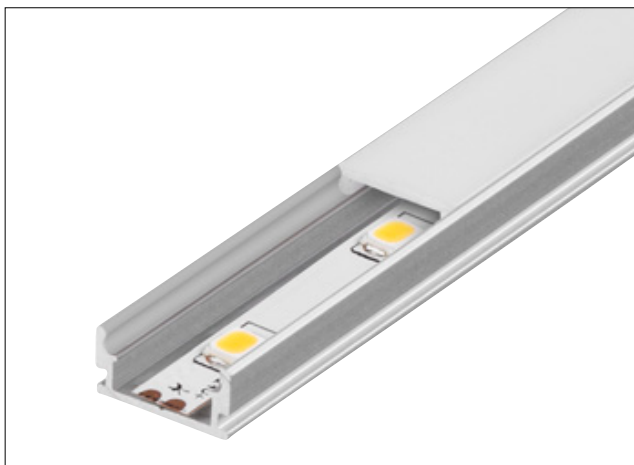
GLENOS Linear-Profil 1107 mit eingeklebtem LED-Strip und Abdeckung
