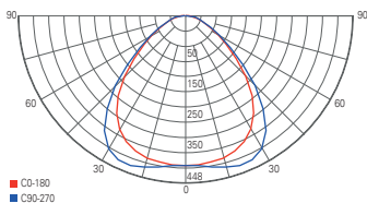
Lichtverteilungskurve 100059
