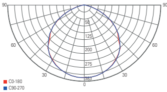
Lichtverteilungskurve 732096
