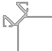
Fliesen-Profil Ecke außen ab Seite 704
