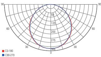
Lichtverteilungskurve 100047
