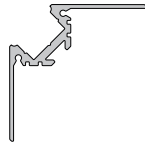
Trockenbau-Profil Ecke Seite 684
