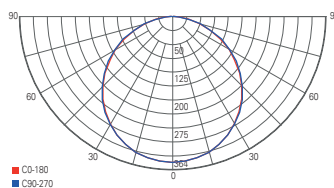
Lichtverteilungskurve 100044
