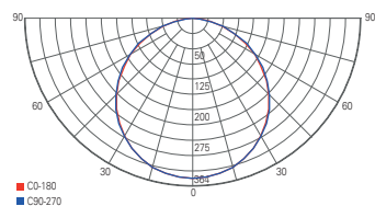
Lichtverteilungskurve 100045
