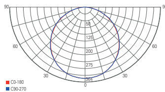
Lichtverteilungskurve 100071
