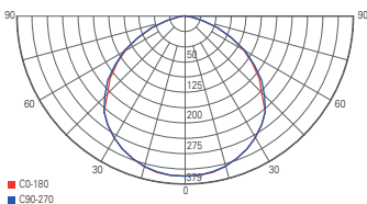
Lichtverteilungskurve 732099
