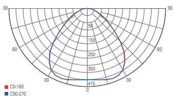
Lichtverteilungskurve 100058
