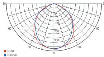
Lichtverteilungskurve 732120
