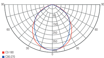
Lichtverteilungskurve 732121
