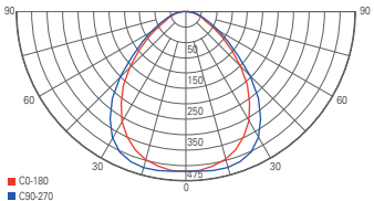
Lichtverteilungskurve 100046
