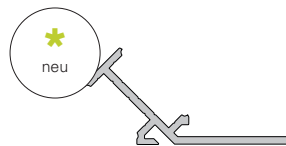
Winkel-Profil Winkel 135° Seite 670
