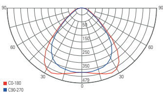
Lichtverteilungskurve 100043
