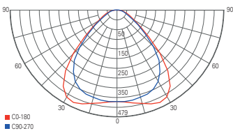
Lichtverteilungskurve 100069
