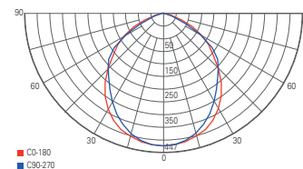
Lichtverteilungskurve 732122
